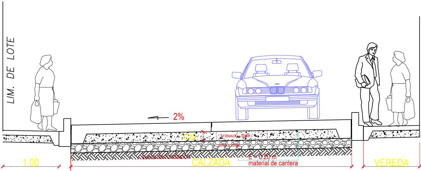
SECCION TIPICA Escala: 1/8
