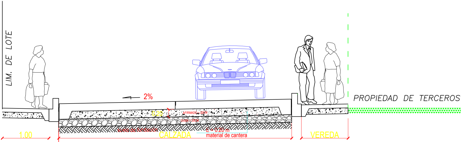
SECCION TIPICA Escala: 1/8
